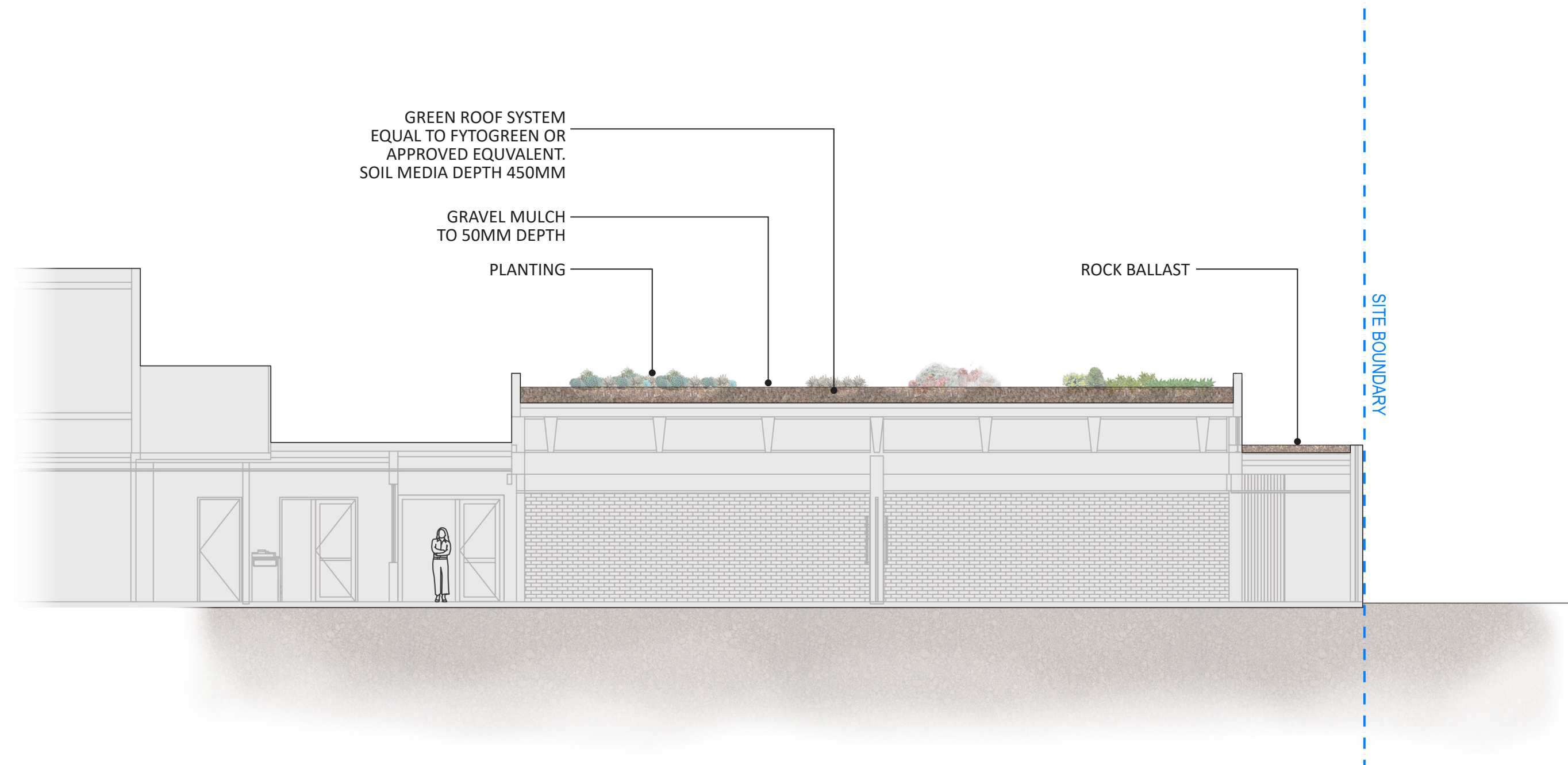
SECTION 01
