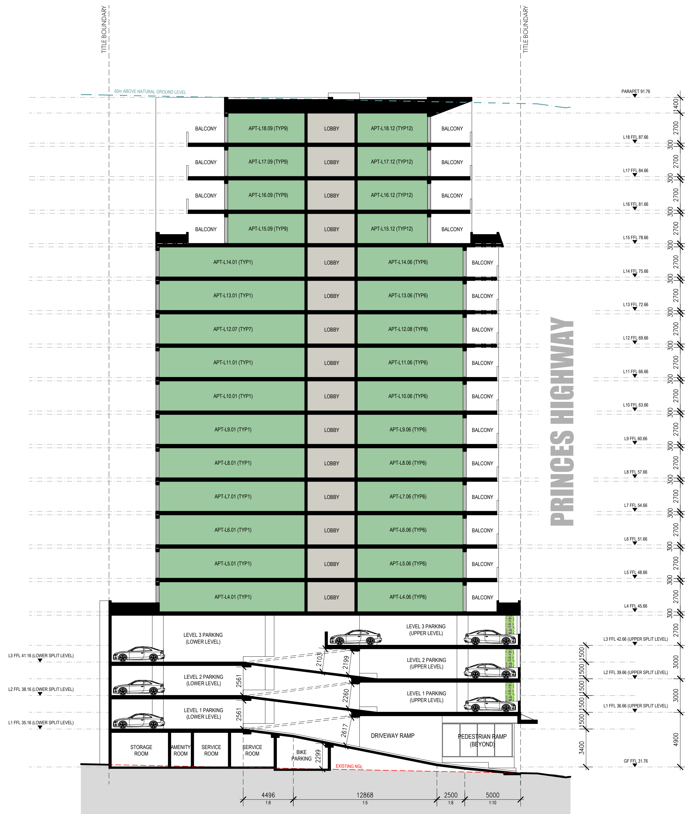
SECTION N A-A 1:200
